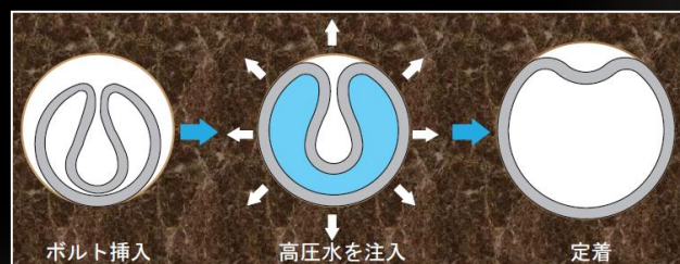
(膨張型ロックボルトの定着機構)
